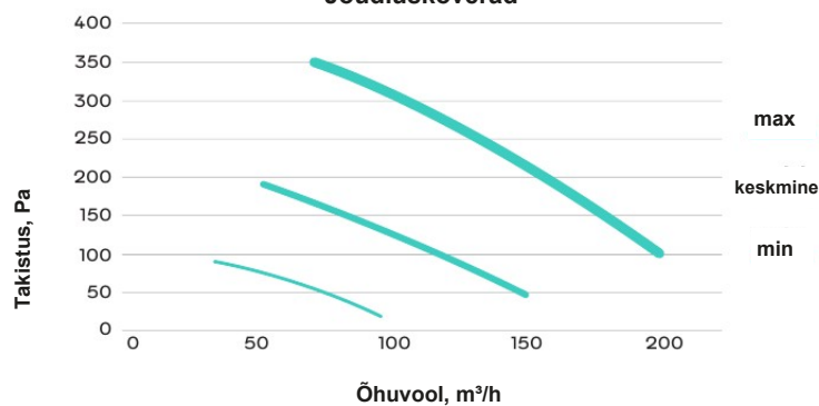
Jõudluskõverad
